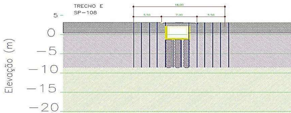
Figura 2. Seção transversal do trecho tratado
