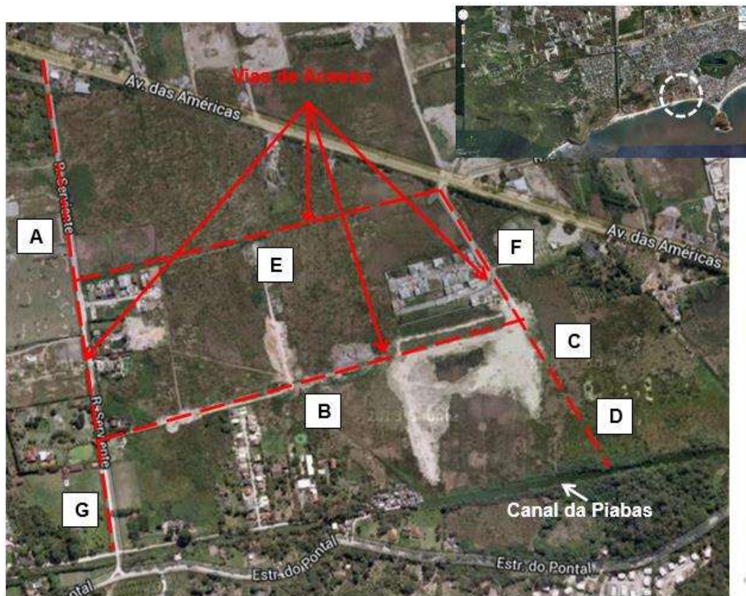
Figura 1. Indicação da localização das vias de acesso e local onde foi realizado os estudos (Fonte Geoinfra, 2015).
